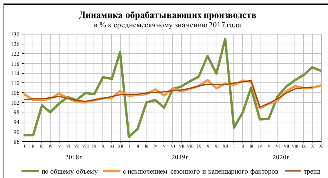
ИНДЕКСЫ ПРОИЗВОДСТВА ПО ОСНОВНЫМ ВИДАМ ОБРАБАТЫВАЮЩИХ ПРОИЗВОДСТВ 1)
